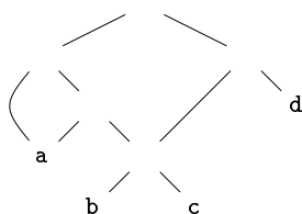
a DAG
